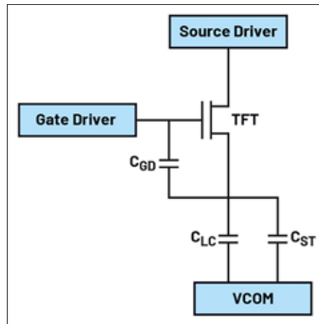
Prinzipieller Aufbau eines herkömmlichen Pixeltreibers
