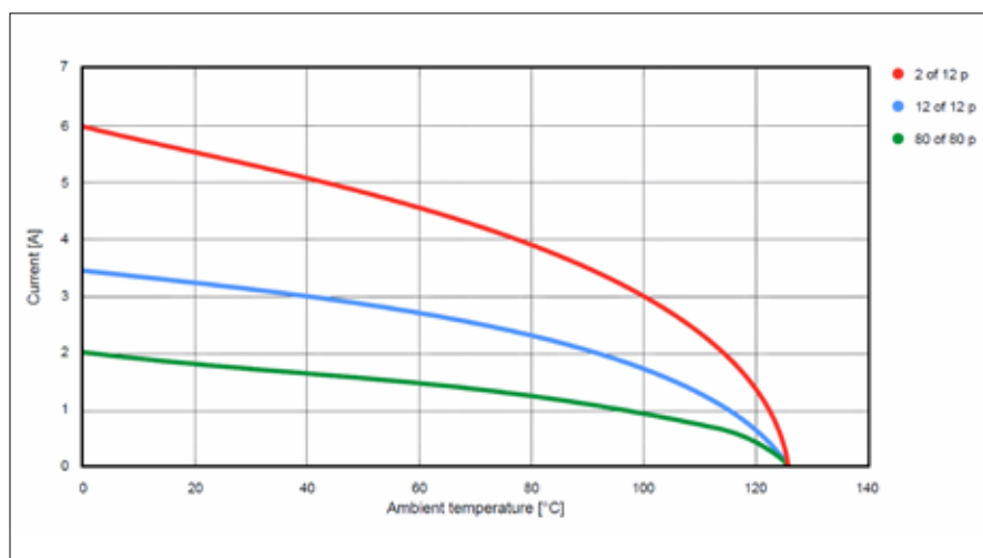
Beispiel Zero8: Stromtragfähigkeit pro Kontakt in Abhängigkeit von Polzahl und Anzahl stromführender Kontakte
