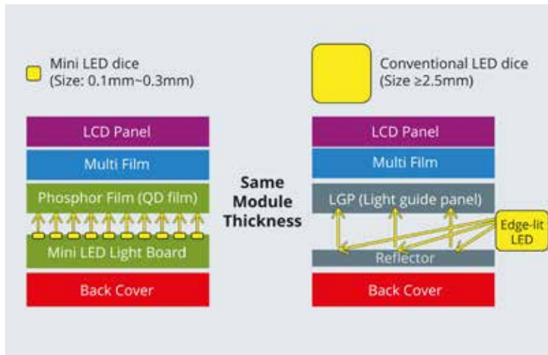
Vergleich: Aufbau Mini-LED und konventionelles Backlight
