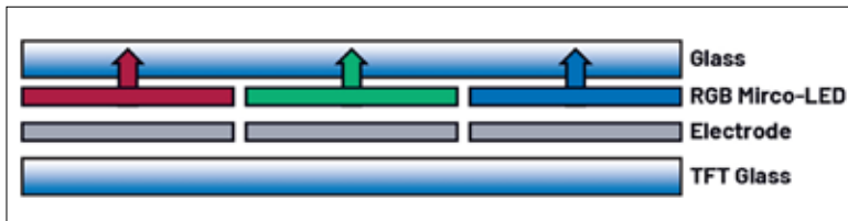
Schematischer Aufbau eines Micro-LED-Displays
