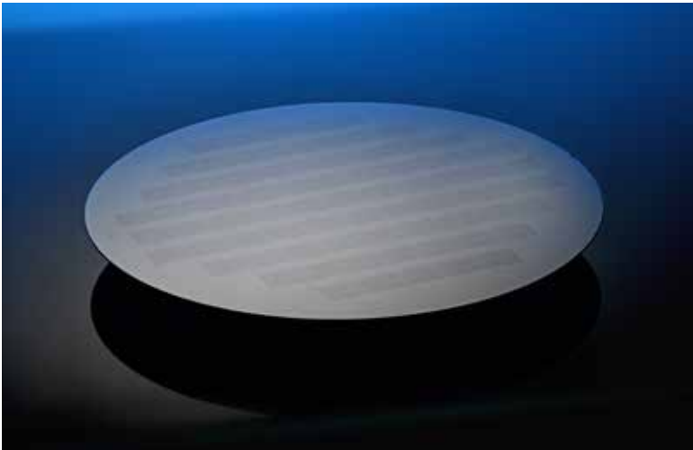
Die selektive Laserkristallisation einer Siliziumschicht auf einem Wafer mit elektrischen Schaltkreisen ermöglicht die integrierte Herstellung von MEMS-Beschleunigungssensoren.
