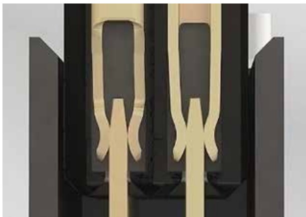
Schematische Details: doppelseitiger Feder- kontakt des One27
