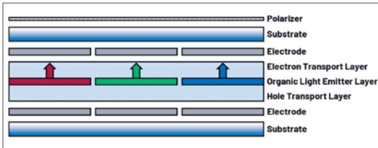
Schematischer Aufbau eines OLED-Displays
