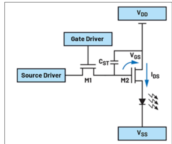
Grundlegender Aufbau eines 2T1C-Pixeltreibers für OLED oder Micro-LED
