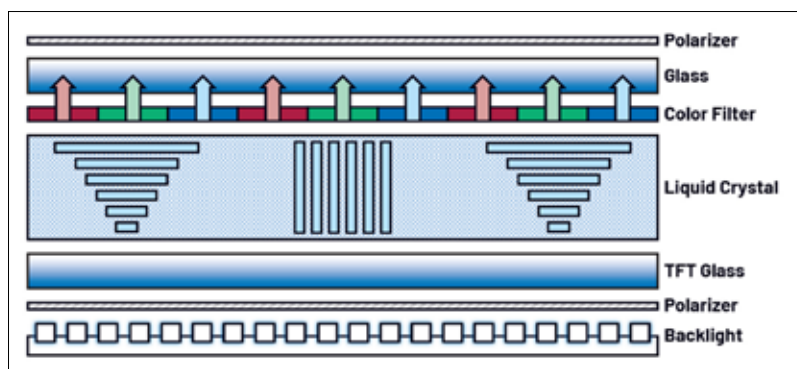
Schematischer Aufbau eines TFT-LCD-Displays
